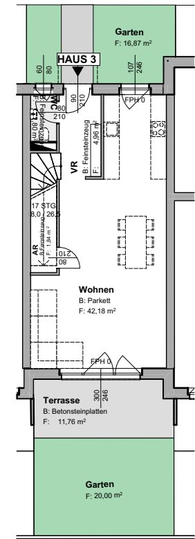
HAUS 3 EG M 1:200
