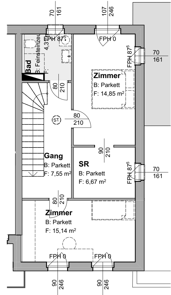
HAUS 3 2.OG M 1:100
