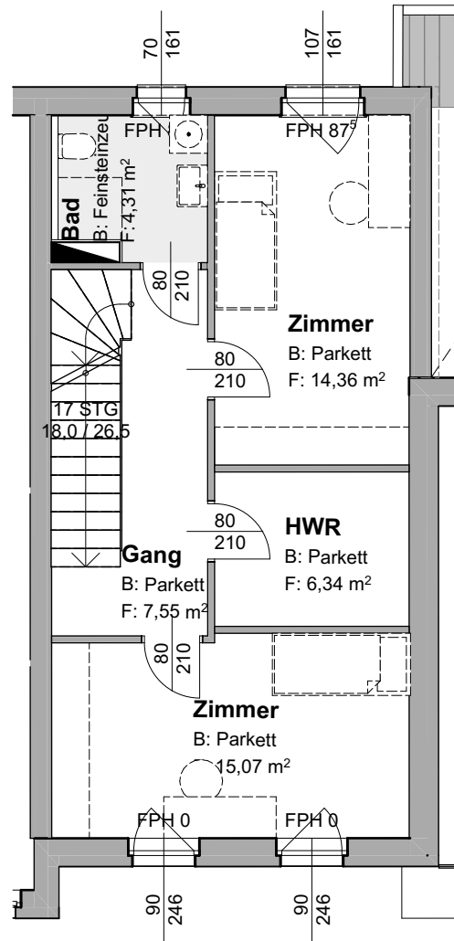
HAUS 3 1.OG M 1:100
