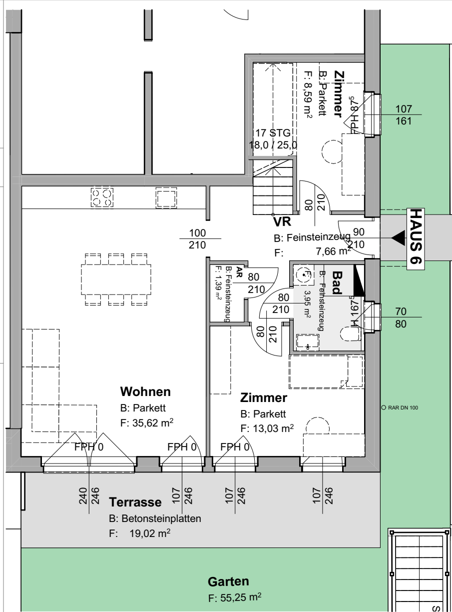
HAUS 6 EG M 1:100
