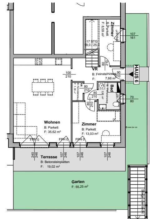
HAUS 6 EG M 1:200
