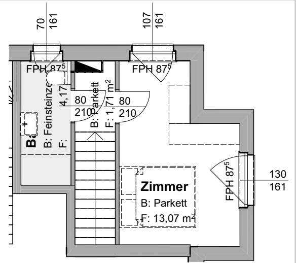
HAUS 6 1.OG M 1:100
