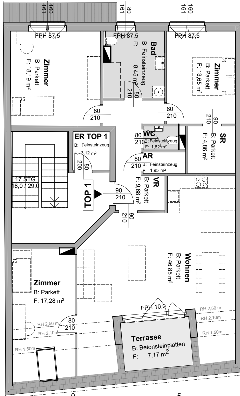
TOP 1 1.OG M 1:100
